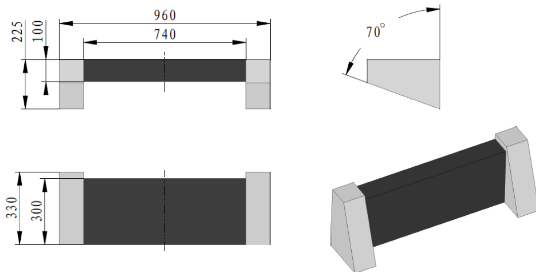
图 20 高墙示意图
