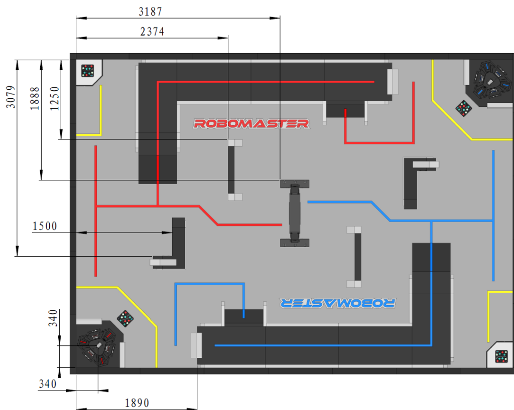
图 5 战场模块定位尺寸图
