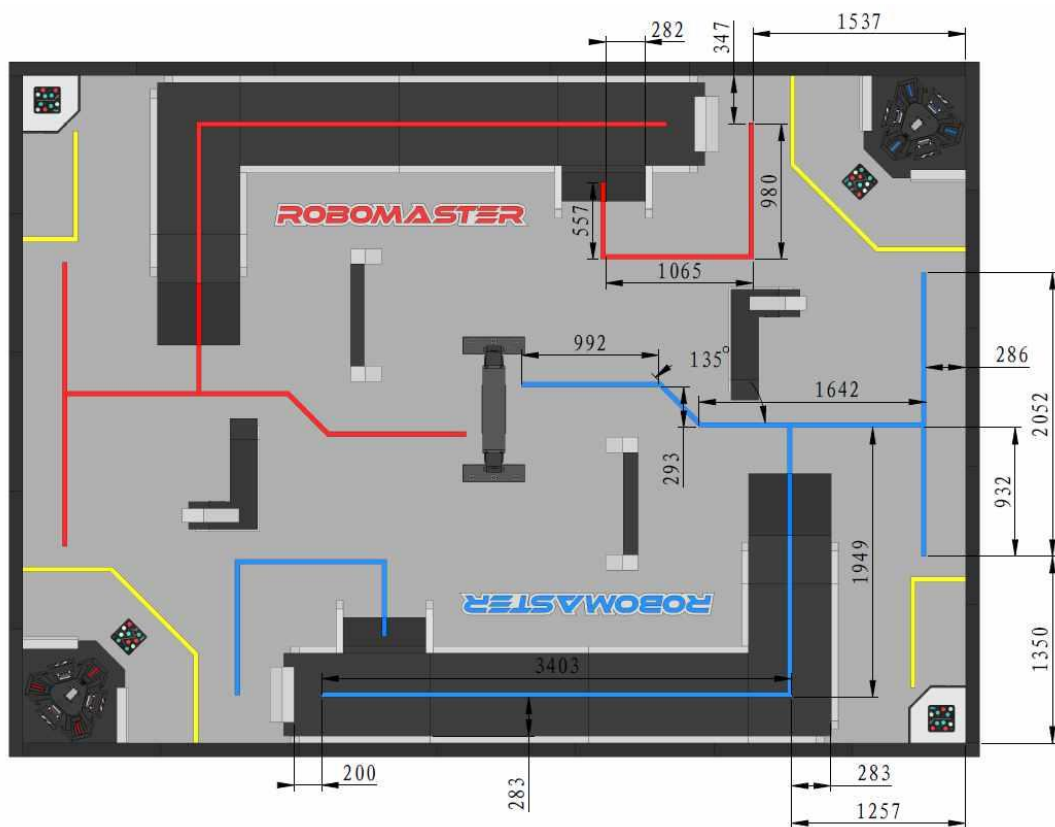
图 29 场地引导线
